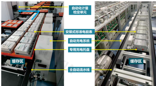
单相流水线
