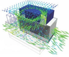
散热功效模拟仿真
